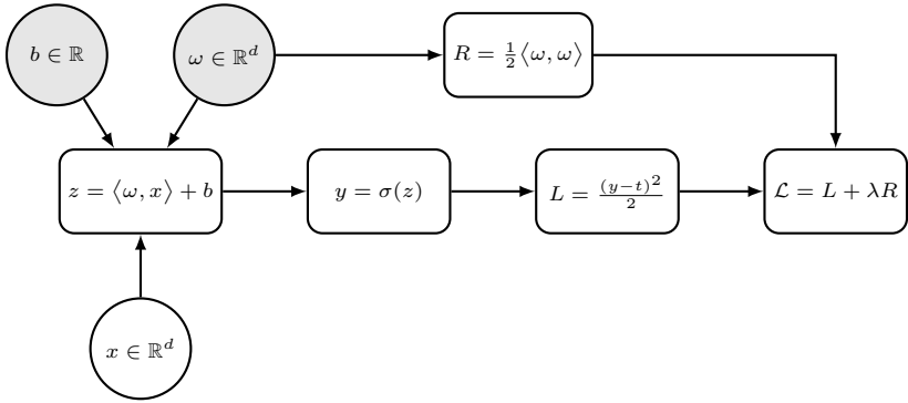
Рис. C1.2: Граф вычислений для логистической регрессии с квадратичной ошибкой и \ell_2 -регуляризацией.
