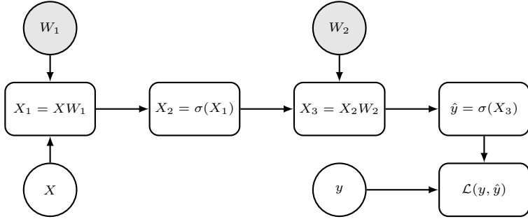
Рис. С1.3: Граф полносвязной нейронной сети.
